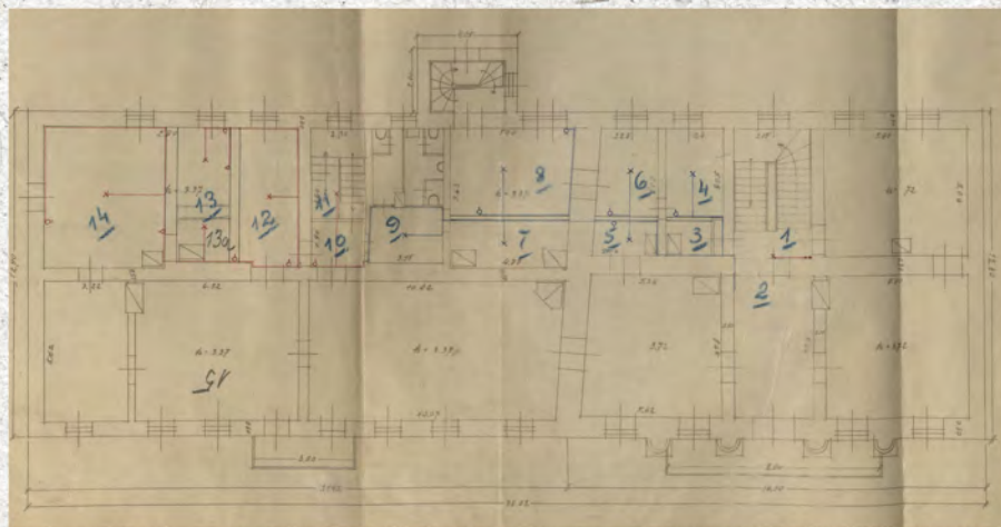
RZUT PIĘTRA GN. WU RATUSZA M. PŁOCKA 1:100
